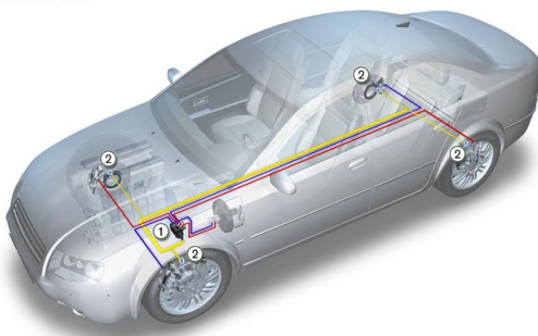
Antiblockiersystem ABS
